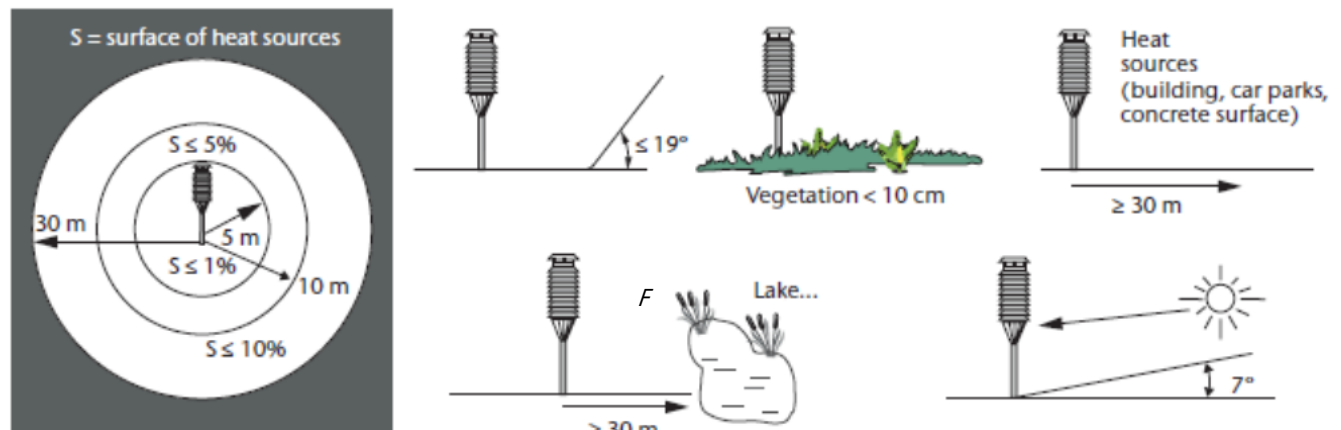
Fig. 4 Temperatura e umidità, criteri per classe 2 (WMO, 2018, Allegato 1.D), pienamente conforme.
