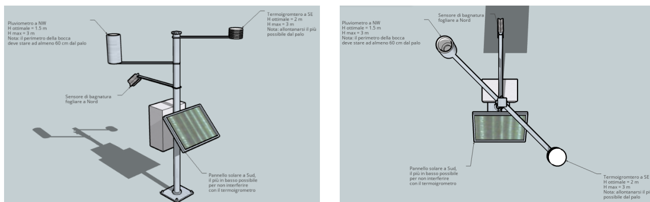
Fig. 13 Esempio di corretta esposizione dei sensori per una stazione che rileva pioggia, temperatura, umidità e bagnatura fogliare.
